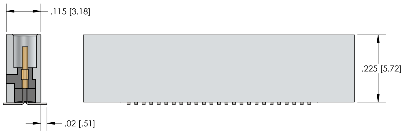
RECEPTACLE (SOCKETS)
