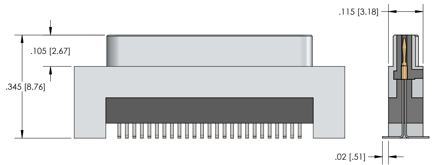
PLUG (PINS)
